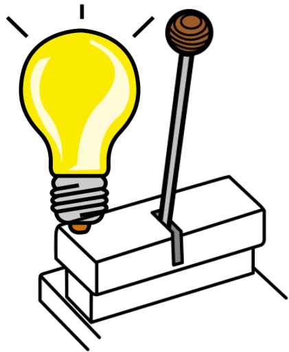
valo - vipu
