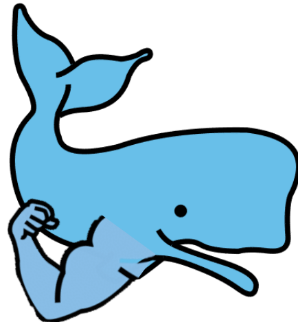
voima - valas
