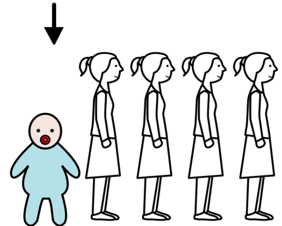
vika - vauva
