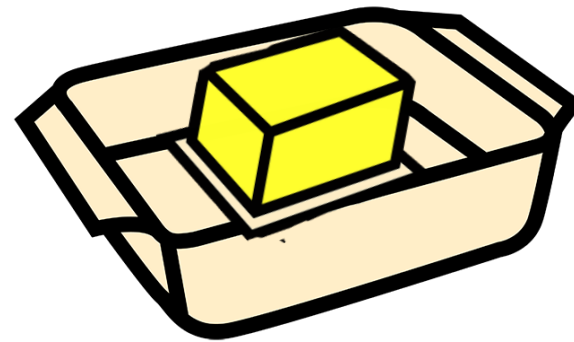
voi - vati
